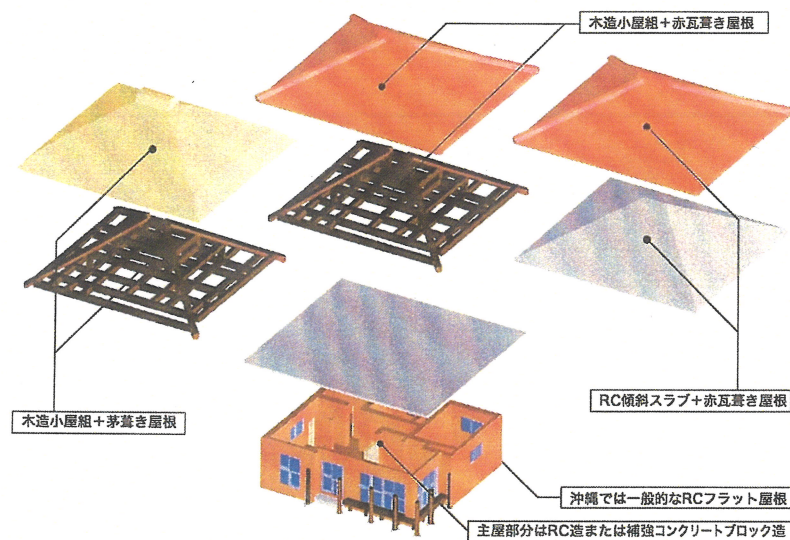
付図-6 修景による屋根葺きの小屋組構造と屋根材の組合せ解説図
